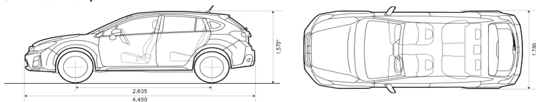
SUBARU XV 2.0i Premium (mm)
