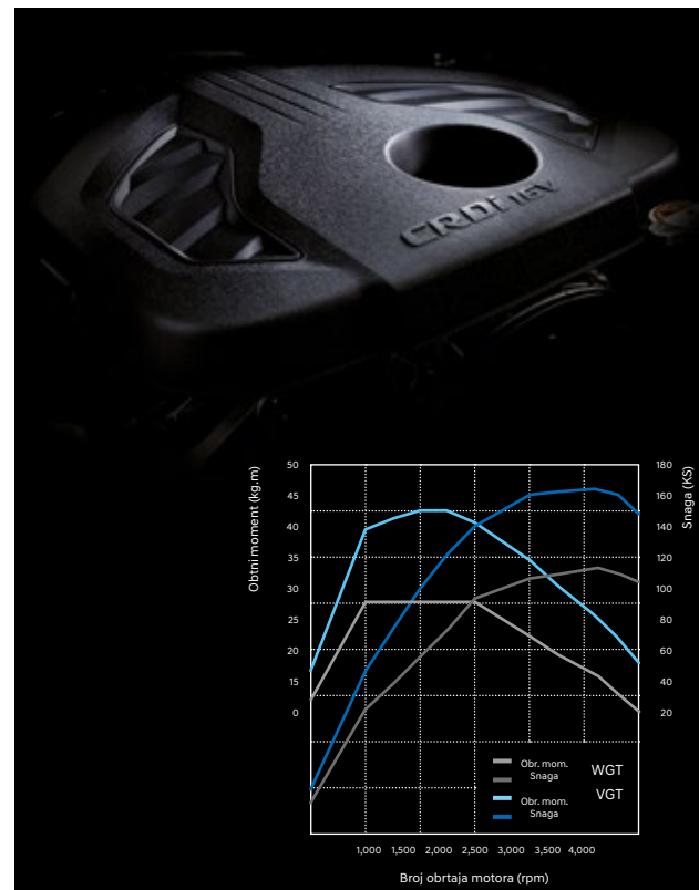
2.5 CRDi dizel motor sa WGT / VGT
